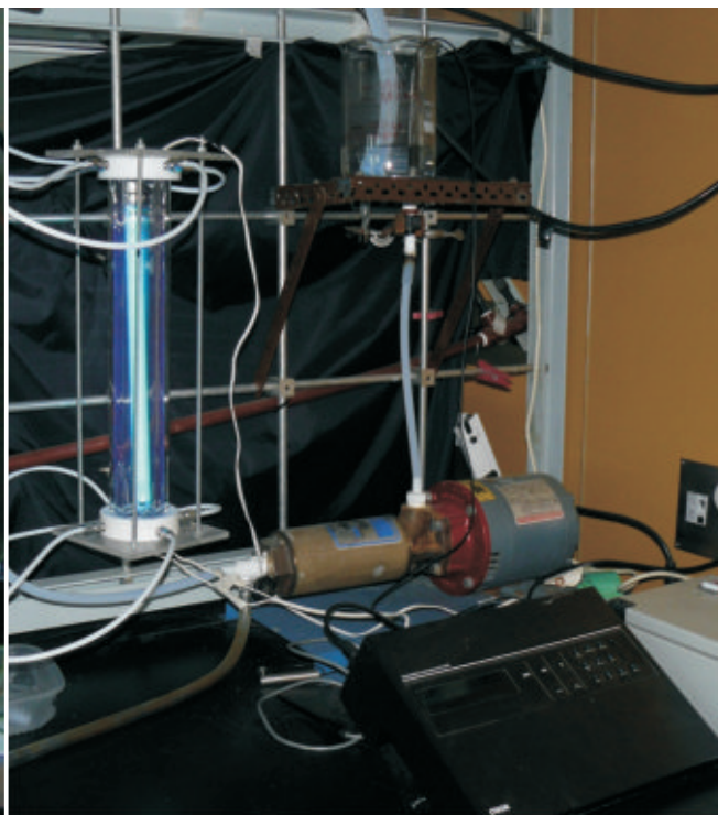
RECICLADO. El programa de gestión y tratamiento de envases de agroquímicos de la UNL se llevan adelante mediante ensayos en un reactor a escala piloto.
