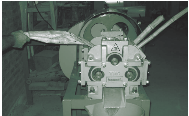
Prototipo de la micro destilería para producir biocombustible.
